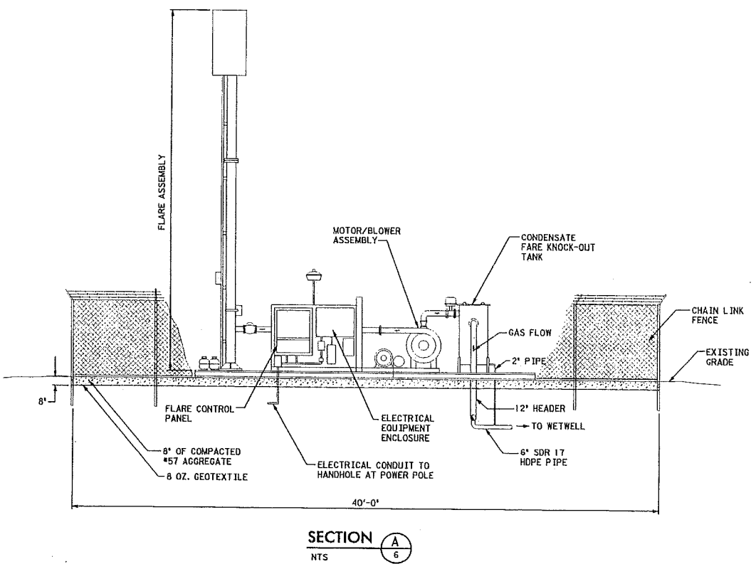
FLARE NTS
