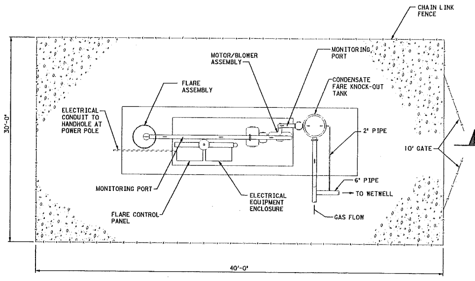
FLARE NTS
